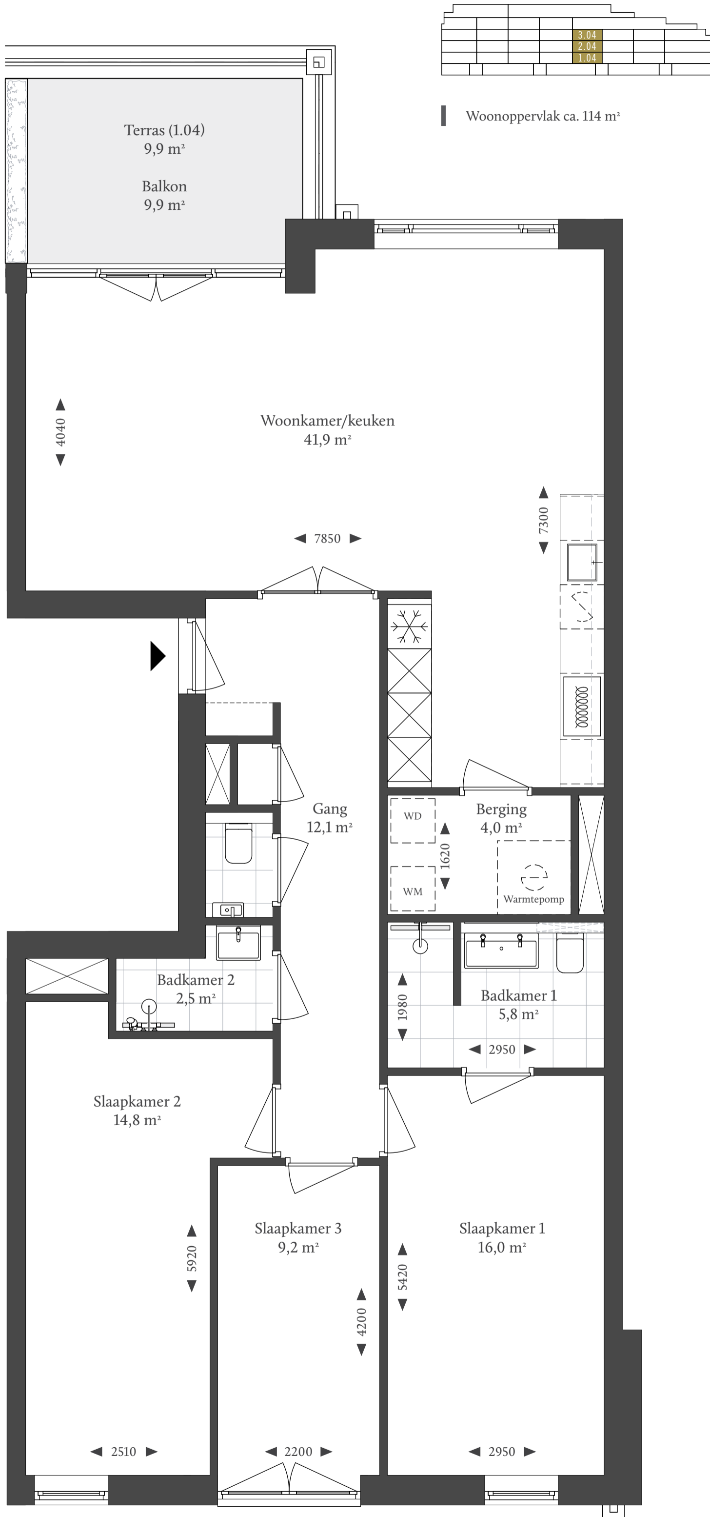
TECHNISCHE PLATTEGROND
